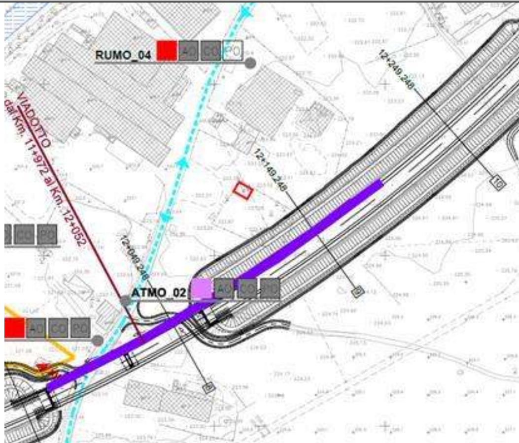
STRALCIO PLANIMETRICO DEL PUNTO DI RILIEVO
