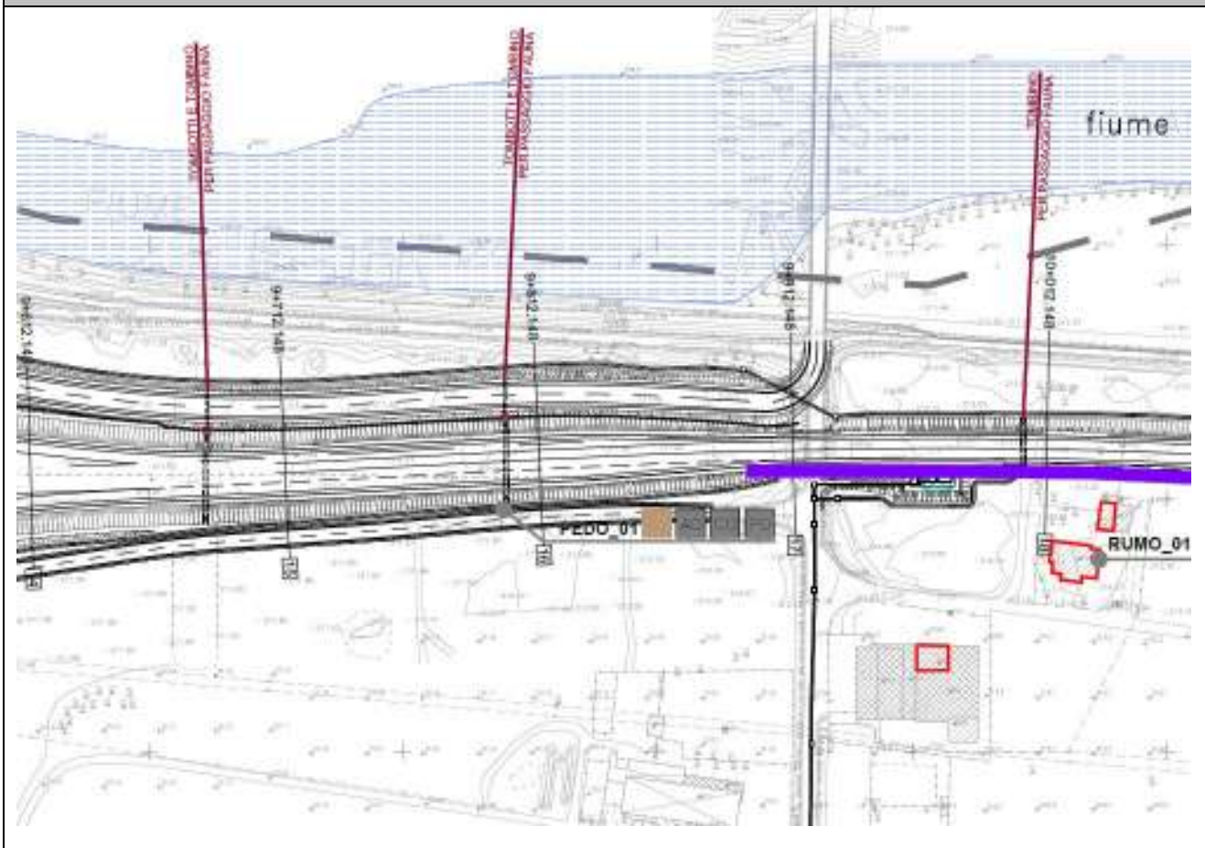
STRALCIO PLANIMETRICO DEL PUNTO DI CAMPIONAMENTO
