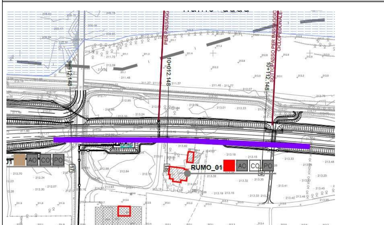
STRALCIO PLANIMETRICO DEL PUNTO DI RILIEVO
